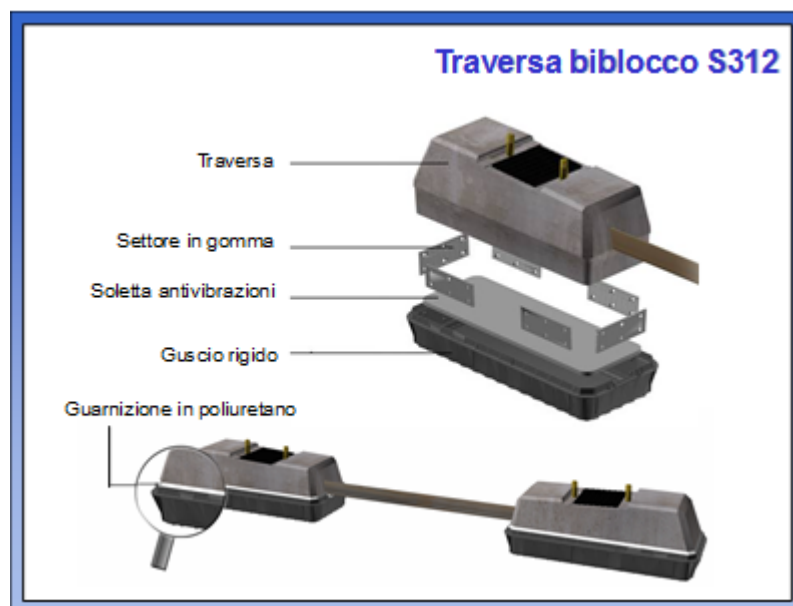
Figura 3 – Traversa biblocco S312
