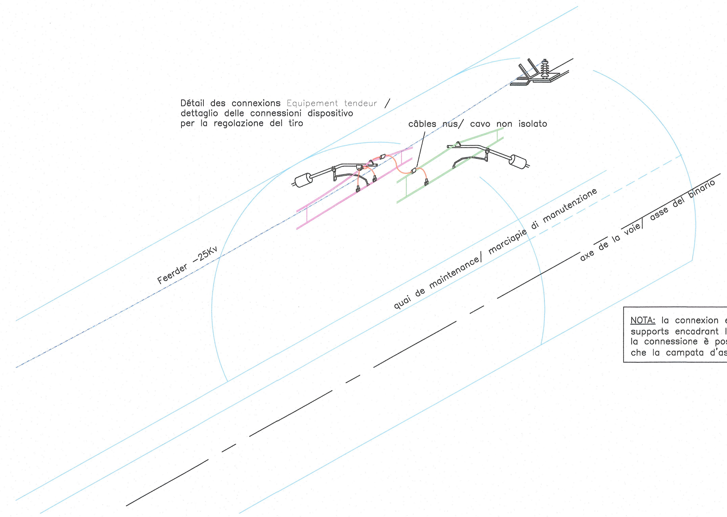
Connexion équipement tendeur / Connessione dispositivo di tensionatura
