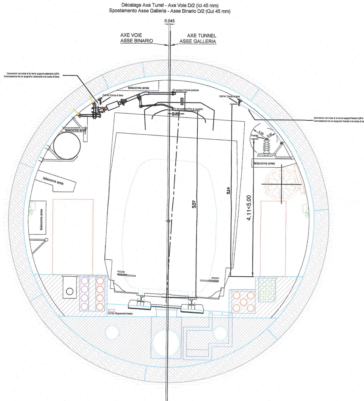
COUPE TYPE COURANTE EN COURBE A GAUCHE (D = 90 mm, DECALAGE 45 mm, R = 3125 m)
