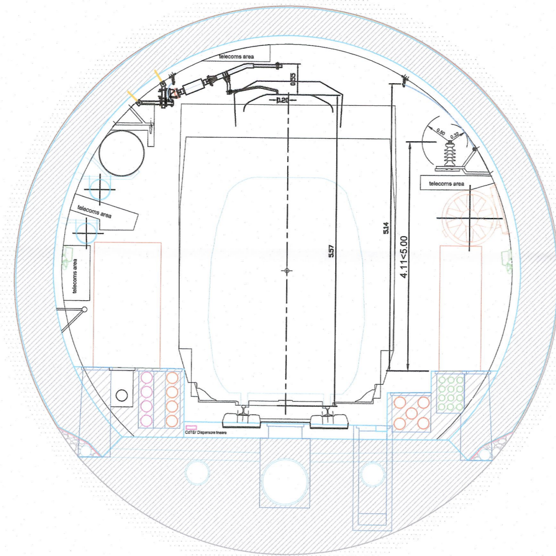
SEZIONE TIPO CORRENTE IN RETTIFILO
