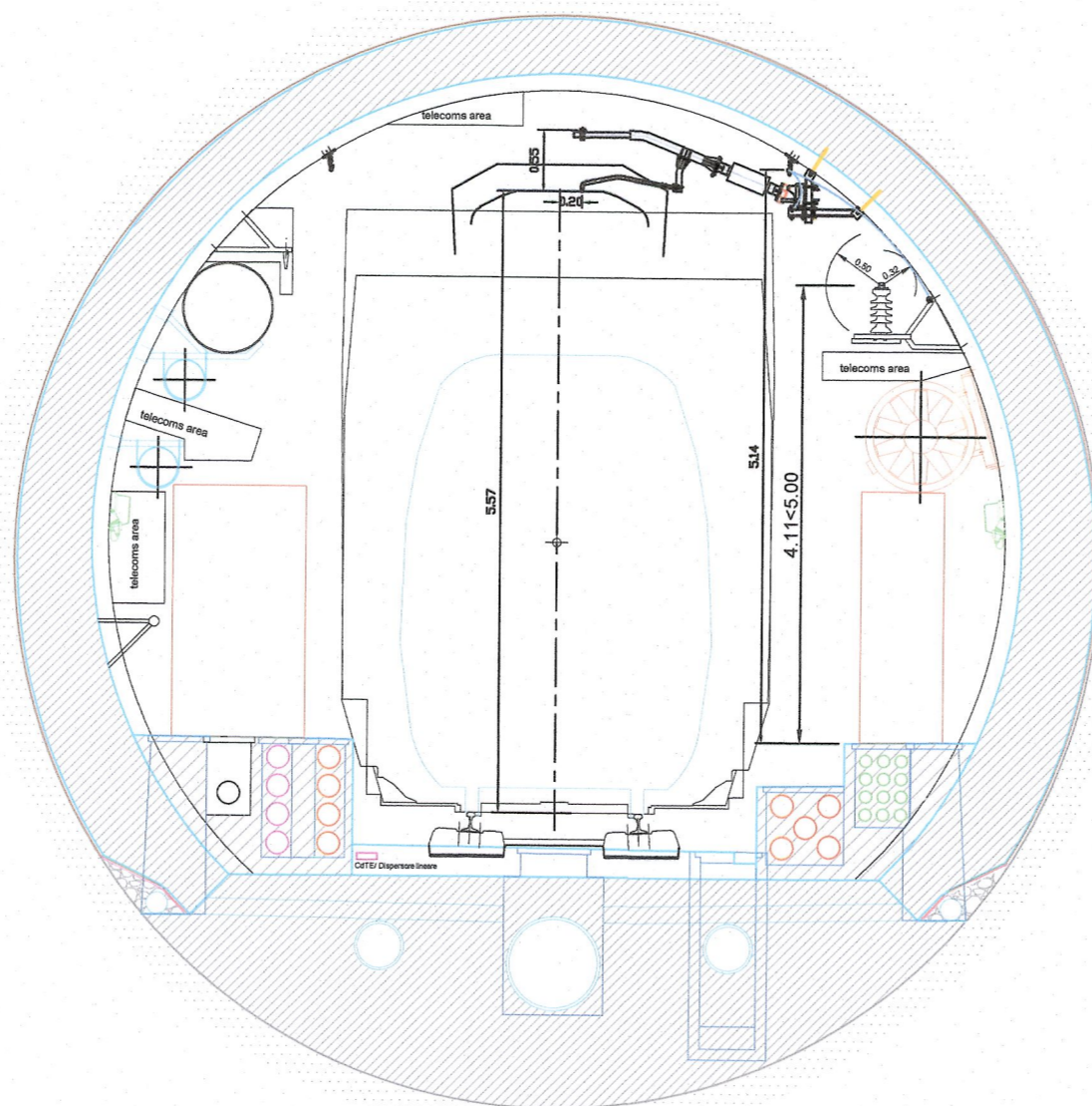
SEZIONE TIPO CORRENTE IN RETTIFILO
