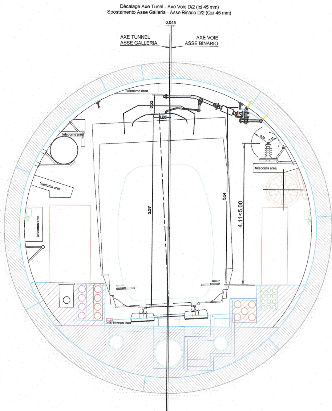
SEZIONE TIPO CORRENTE IN CURVA A SINISTRA (D = 90 mm, SPOSTAMENTO 45 mm, R = 3125 m)
