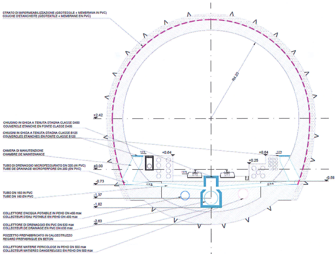
Figure 10 – Sezione tipo del drenaggio delle acque freatiche per scavo tradizionale
