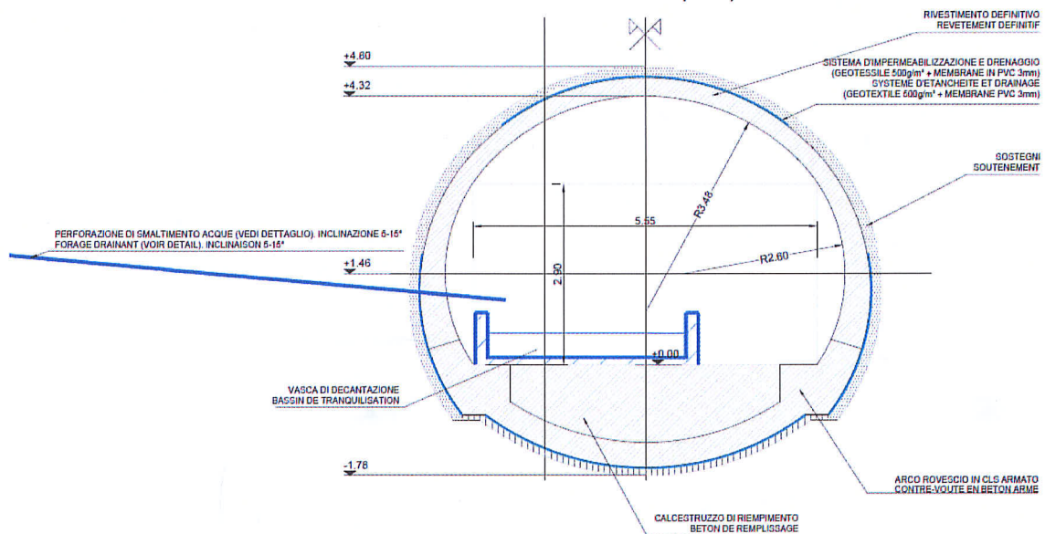
Figura 14 – Sistema di captazione delle acque calde potenzialmente potabili. Sezione trasversale della nicchia
