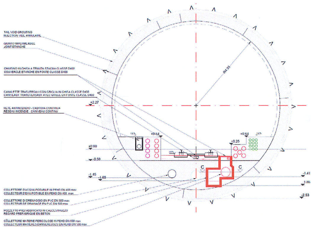
Figura 16 – Sezione trasversale del sistema di raccolta dei liquidi pericolosi – Caso di rettilo e curva a destra
