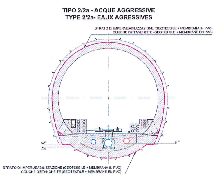
Figure 2 – Impermeabilizzazione di tipo 2/2a per scavo tradizionale
