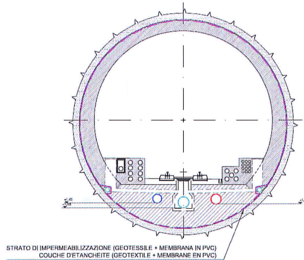
Figure 7 – Impermeabilizzazione di tipo 5/5a per scavo con TBM aperta
