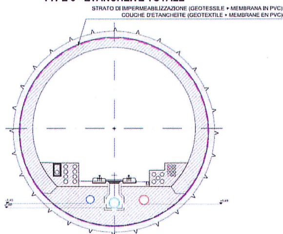
Figura 4 – Impermeabilizzazione di tipo 3 per scavo con TBM aperta
