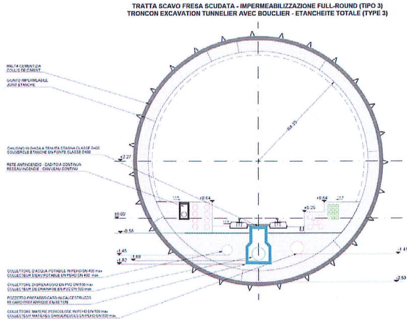
Figure 5 – Impermeabilizzazione di tipo 3 per scavo con TBM scudata
