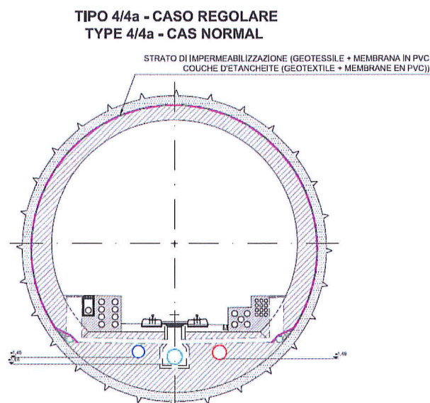
Figura 6 – Impermeabilizzazione di tipo 4/4a per scavo con TBM aperta
