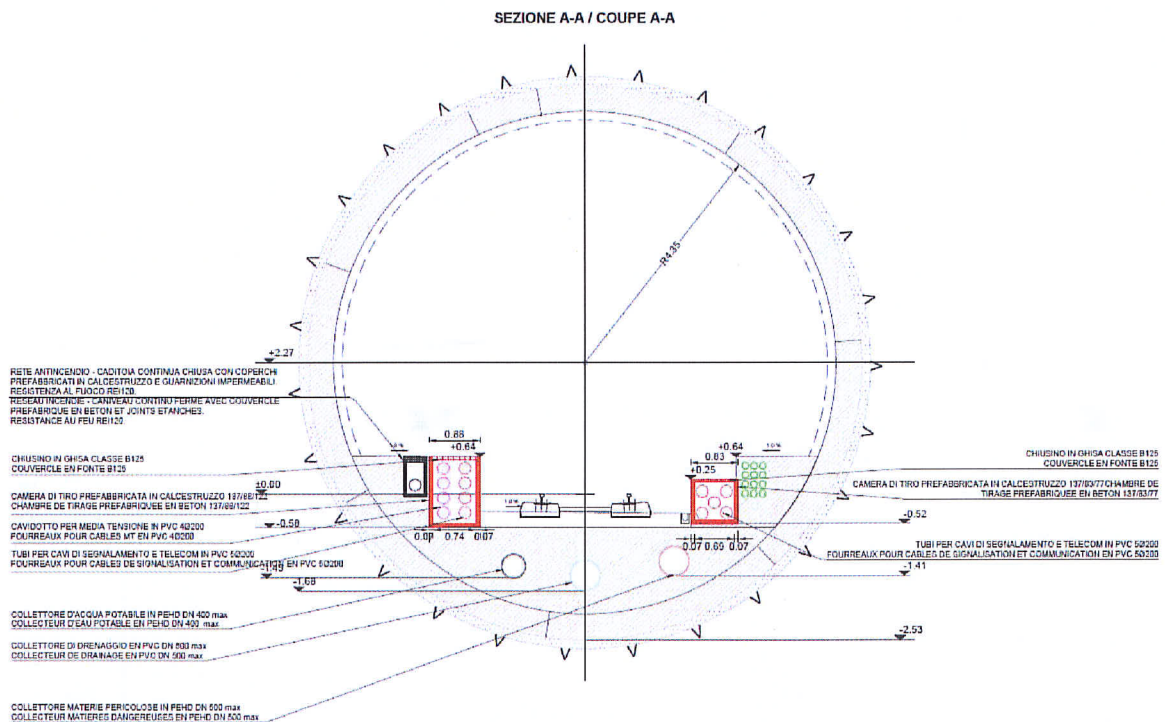
Figure 21 – Sezione trasversale A-A delle camere di tiro e della rete antincendio
