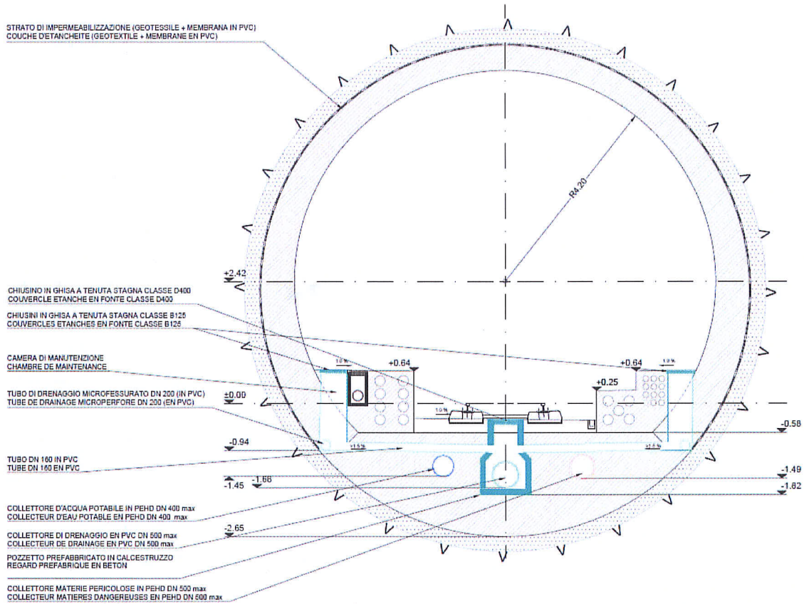
Figure 11 – Sezione tipo del drenaggio delle acque freatiche per scavo con TBM aperta
