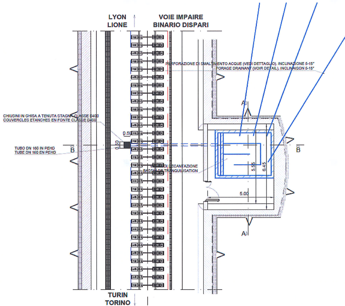
Figura 12 – Sistema di captazione delle acque calde potenzialmente potabili. Planimetria
