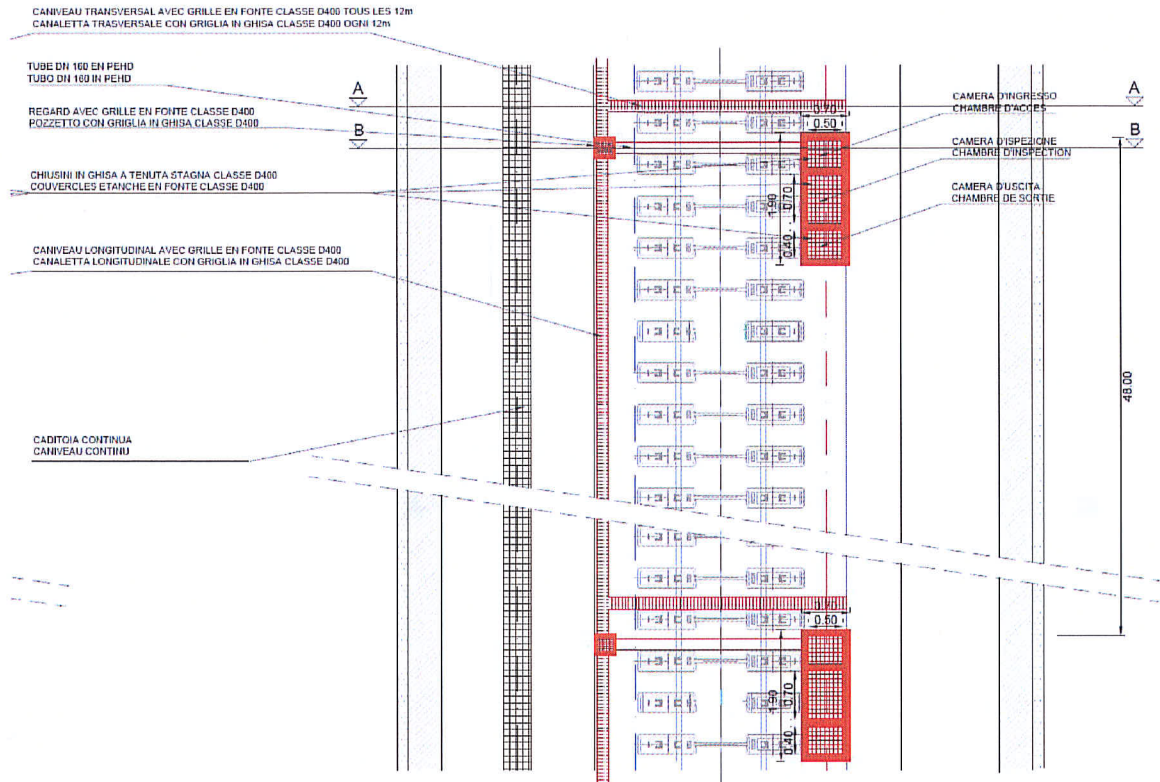
Figura 17 – Planimetria del sistema di raccolta dei liquidi pericolosi – Caso di curva a sinistra
