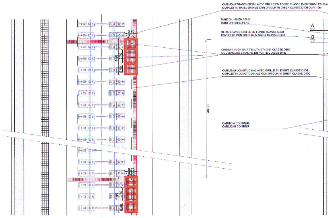
Figura 15 – Planimetria del sistema di raccolta dei liquidi pericolosi – Caso di rettilo e curva a destra
