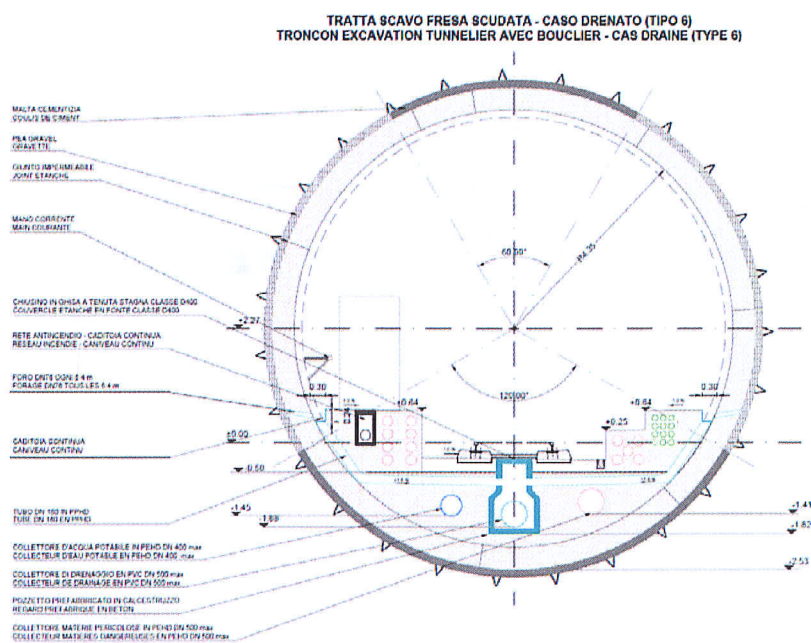
Figure 9 – Sezione tipo del sistema di drenaggio delle acque freatiche per scavo con TBM scudata
