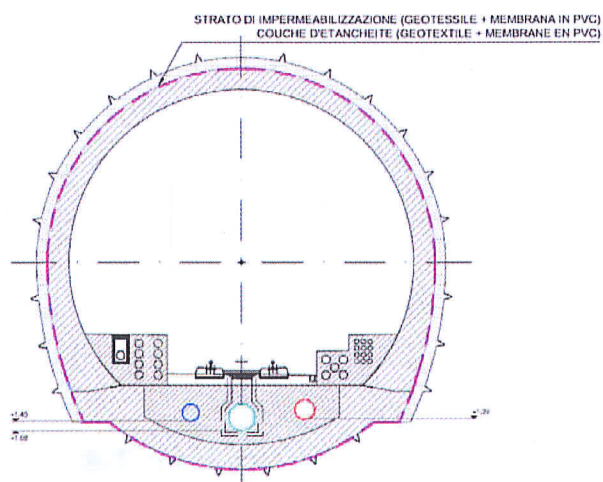
Figura 3 – Impermeabilizzazione di tipo 3 per scavo tradizionale
