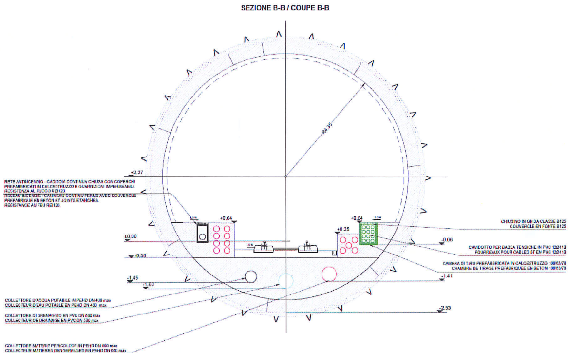
Figure 22 – Sezione trasversale B-B delle camere di tiro e della rete antincendio
