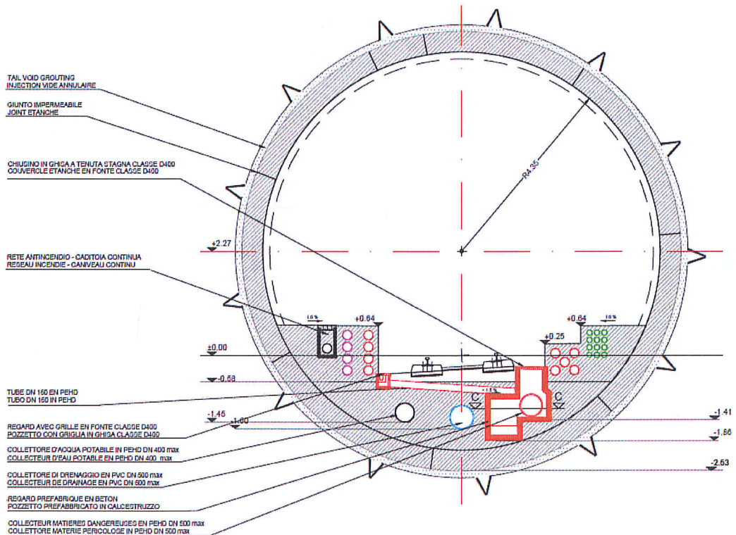
Figura 18 – Sezione trasversale del sistema di raccolta dei liquidi pericolosi – Caso di curva a sinistra
