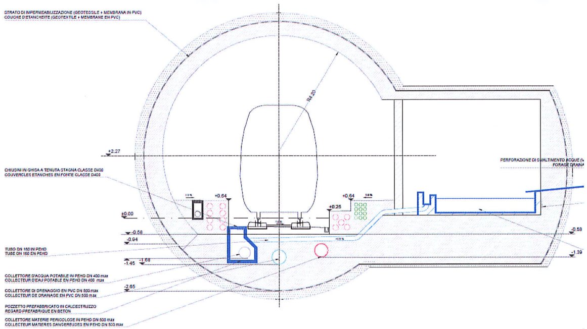
Figura 13 – Sistema di captazione delle acque calde potenzialmente potabili. Sezione longitudinale della nicchia
