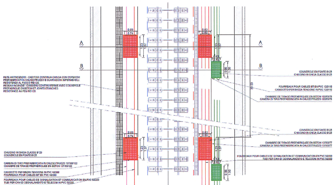
Figure 20 – Planimetria delle camere di tiro e della rete antincendio
