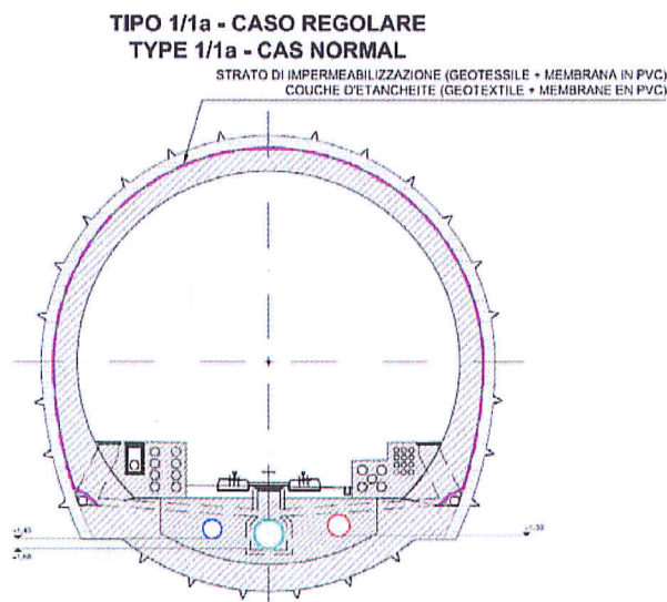
Figura 1 – Impermeabilizzazione di tipo 1/1a per scavo tradizionale
