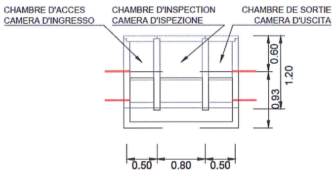
Figura 19 – Dettaglio dei sifoni tagliafuoco
