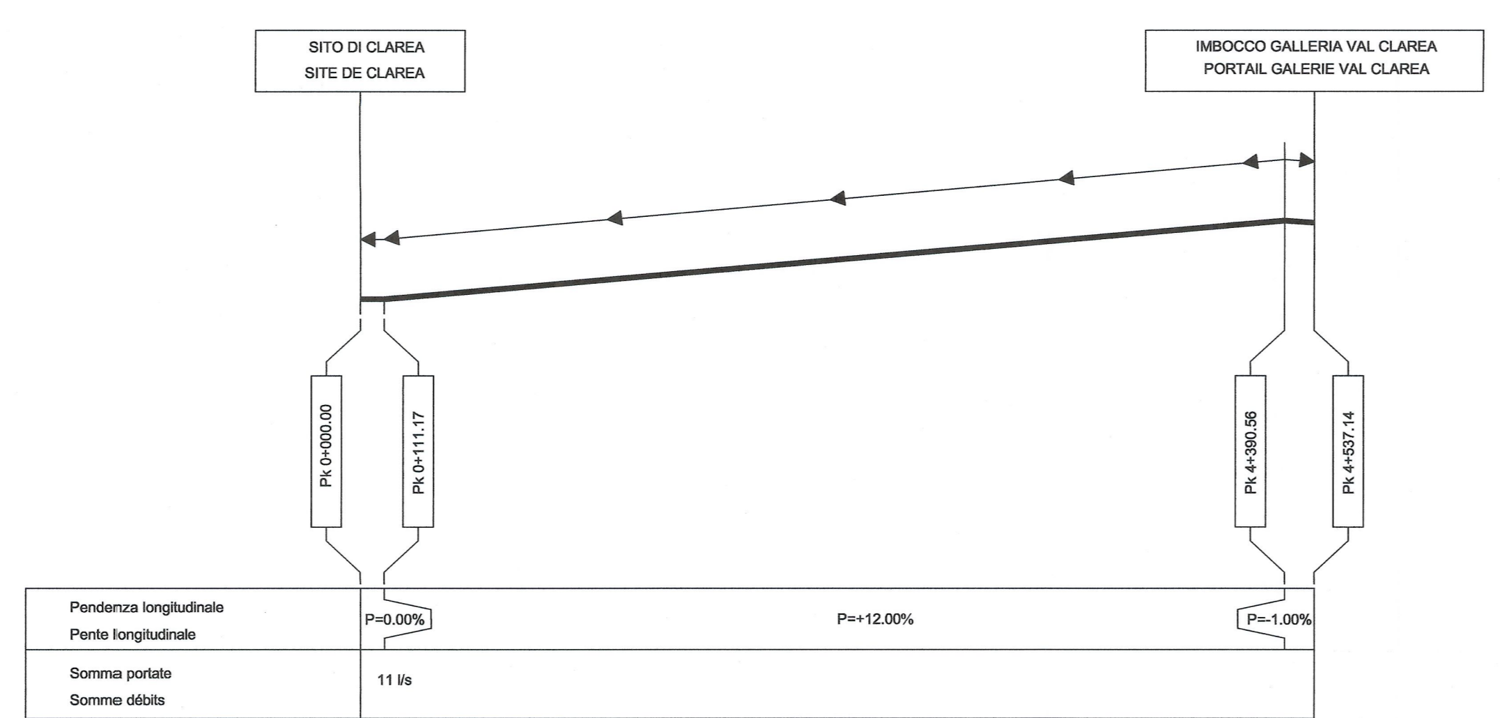
SEZIONE SCHEMATICA LONGITUDINALE / COUPE SCHEMATIQUE LONGITUDINALE
