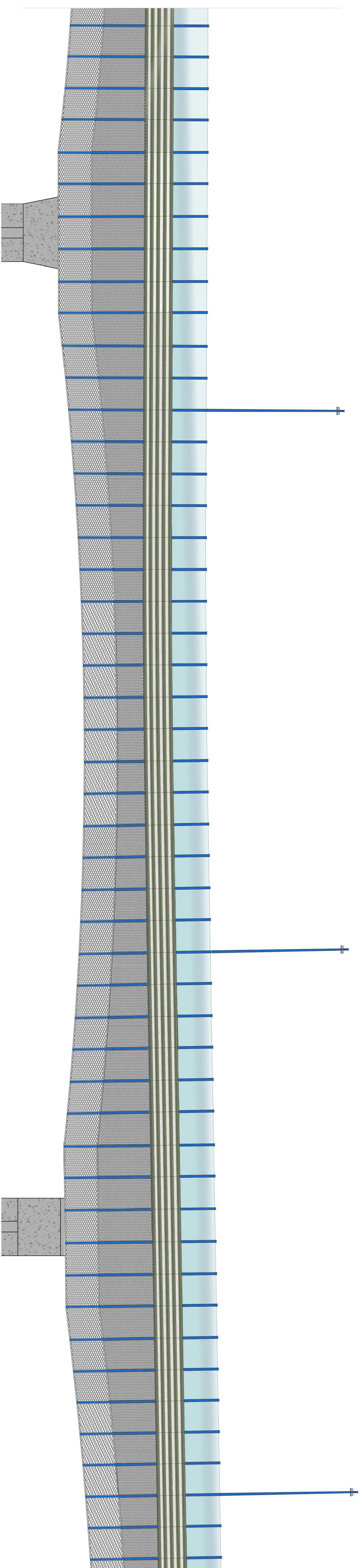
Stralcio Prospetto Sud Scala 1:100
