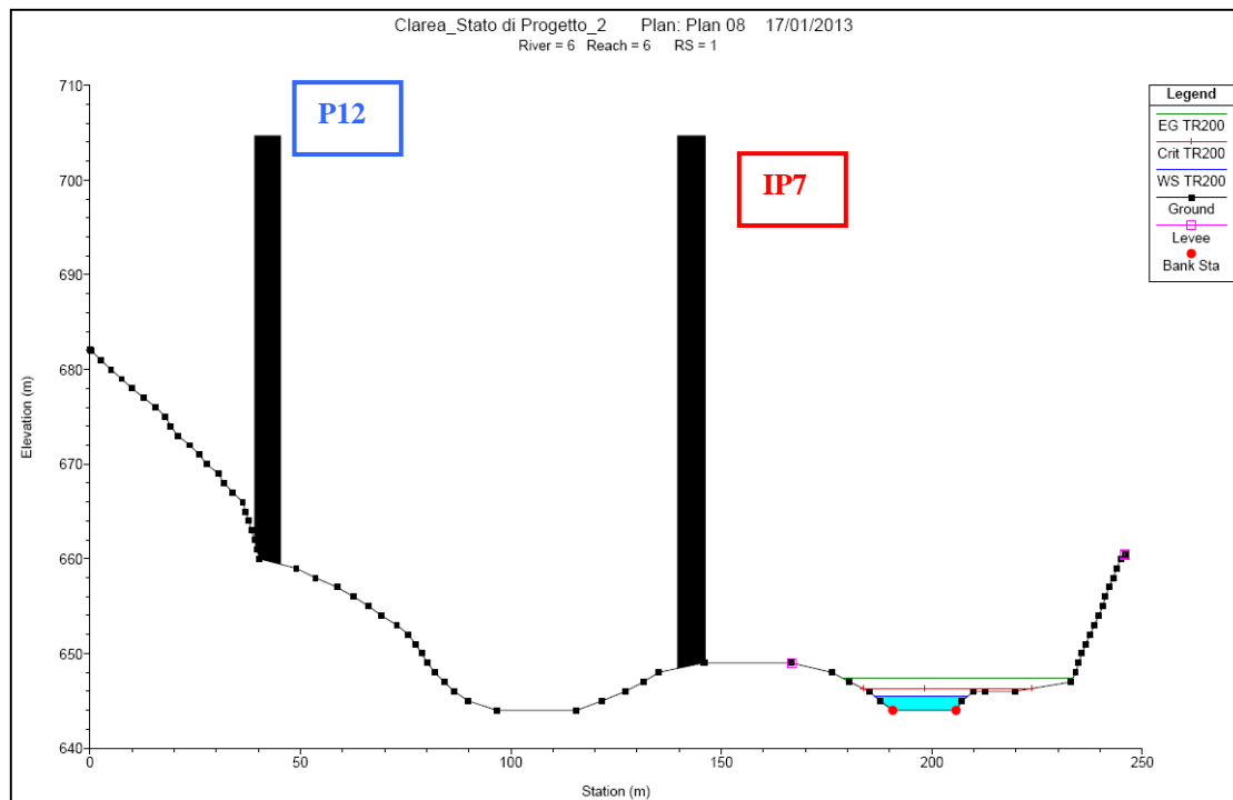
Fig. 17 – Sezione idraulica RS1
