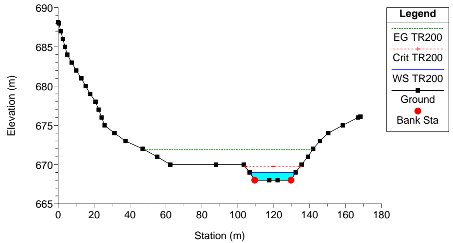
Clarea_Stato attuale Plan: Plan 08 21/01/2013 River = 6 Reach = 6 RS = 24
