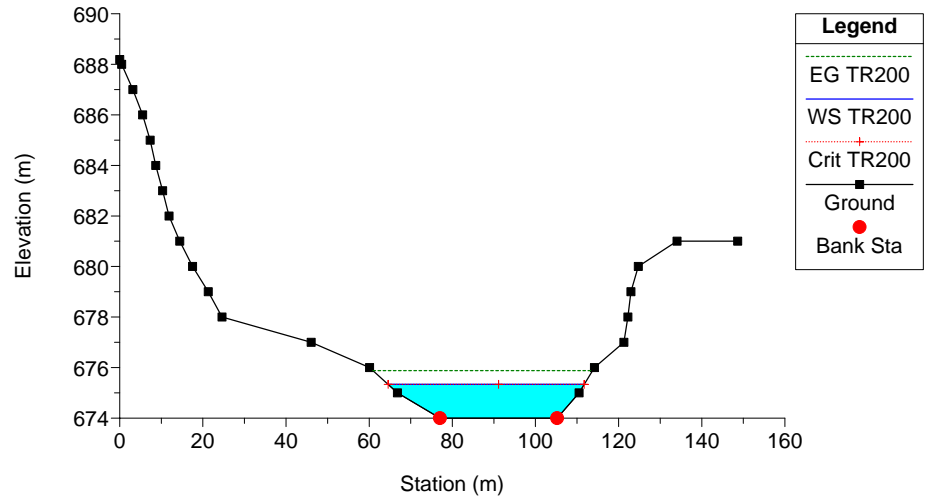
Clarea_Stato di Progetto_2 Plan: Plan 11 21/01/2013 River = 6 Reach = 6 RS = 29
