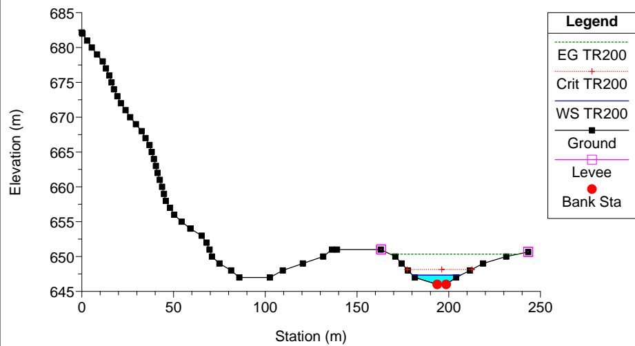
Clarea_Stato di Progetto_2 Plan: Plan 11 21/01/2013 River = 6 Reach = 6 RS = 4
