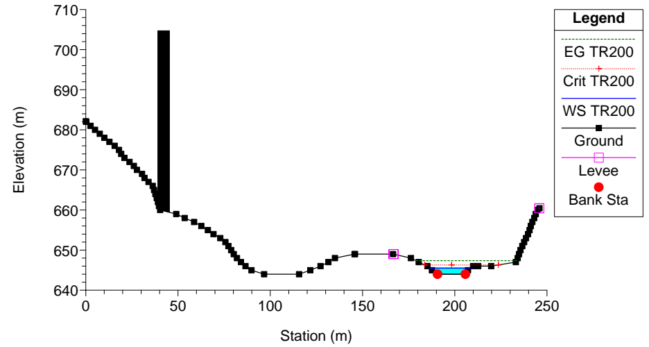
Clarea_Stato attuale Plan: Plan 08 21/01/2013 River = 6 Reach = 6 RS = 1
