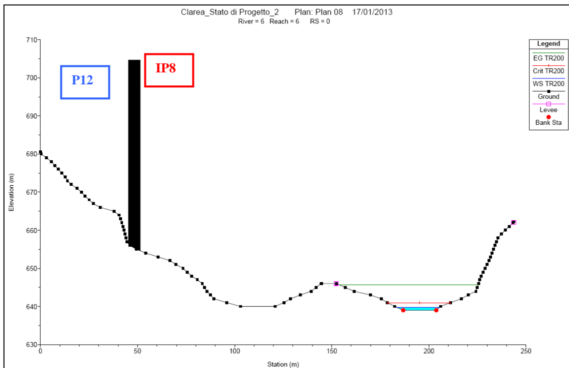
Fig. 16 – Sezione idraulica RS0
