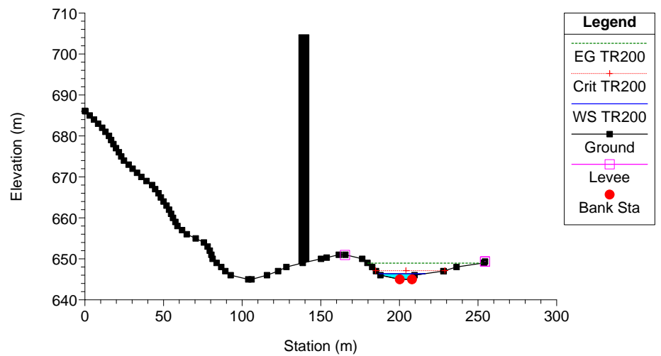
Clarea_Stato attuale Plan: Plan 08 21/01/2013 River = 6 Reach = 6 RS = 3
