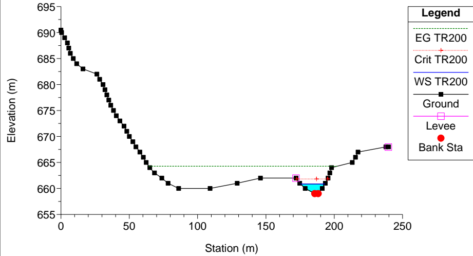
Clarea_Stato di Progetto_2 Plan: Plan 11 21/01/2013 River = 6 Reach = 6 RS = 17
