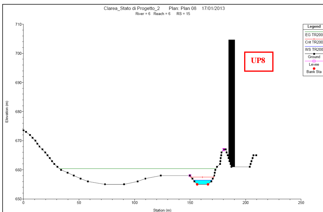
Fig. 19 – Sezione idraulica RS15
