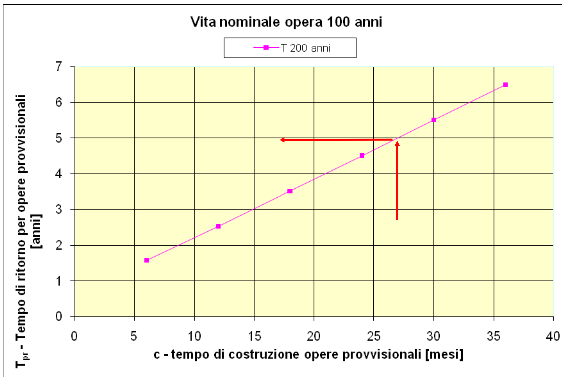
Fig. 21 –Variazione del tempo di ritorno per la verifica delle opere provvisionali in funzione della vita dell'opera ( V ) e del tempo di costruzione ( c ).
