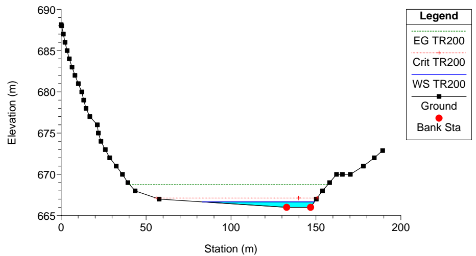
Clarea_Stato attuale Plan: Plan 08 21/01/2013 River = 6 Reach = 6 RS = 24
