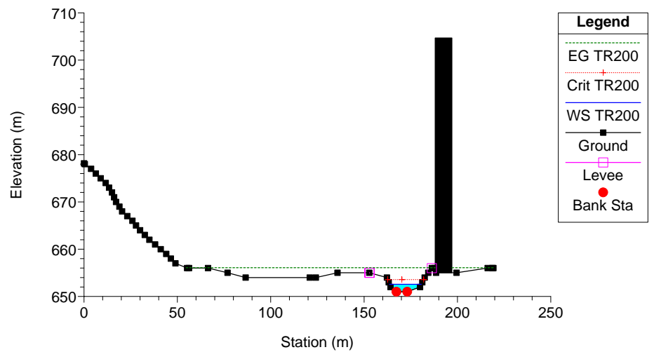
Clarea_Stato attuale Plan: Plan 08 21/01/2013 River = 6 Reach = 6 RS = 10
