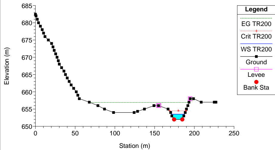
Clarea_Stato attuale Plan: Plan 08 21/01/2013 River = 6 Reach = 6 RS = 11
