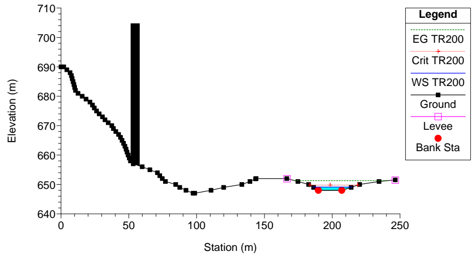
Clarea_Stato attuale Plan: Plan 08 21/01/2013 River = 6 Reach = 6 RS = 3
