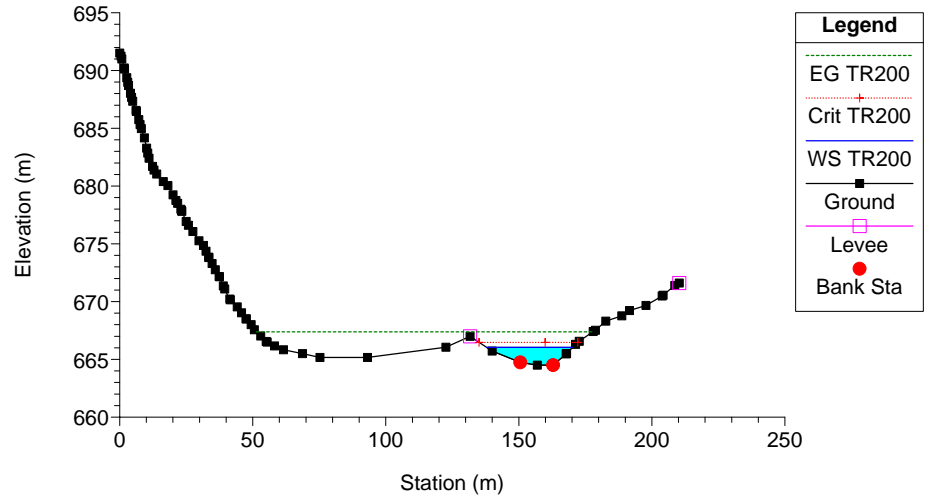
Clarea_Stato di Progetto_2 Plan: Plan 11 21/01/2013 River = 6 Reach = 6 RS = 20
