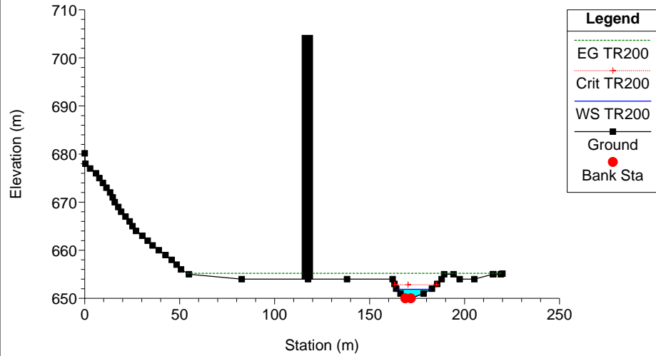
Clarea_Stato attuale Plan: Plan 08 21/01/2013 River = 6 Reach = 6 RS = 8
