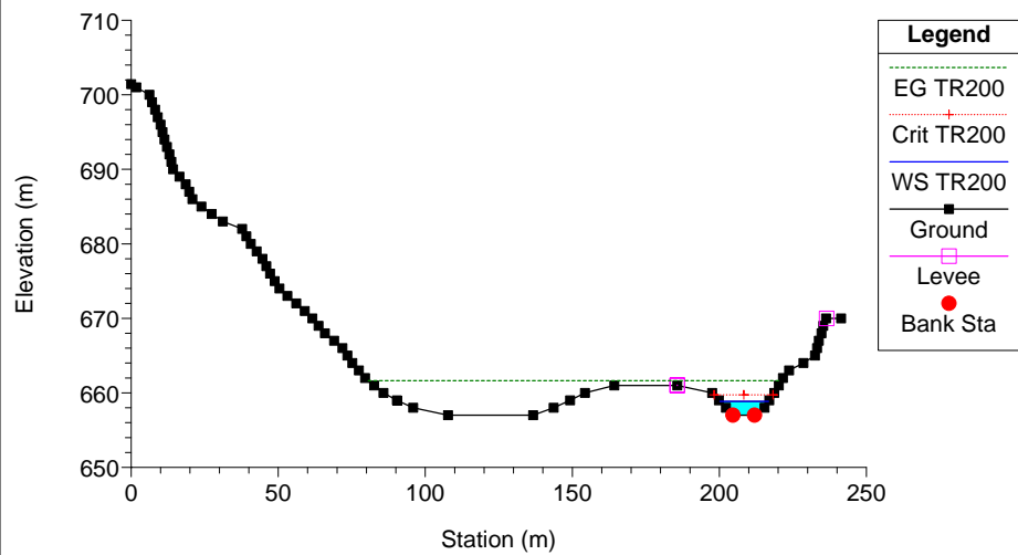
Clarea_Stato attuale Plan: Plan 08 21/01/2013 River = 6 Reach = 6 RS = 17
