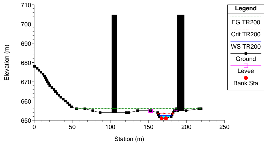
Clarea_Stato di Progetto_2 Plan: Plan 11 21/01/2013 River = 6 Reach = 6 RS = 10
