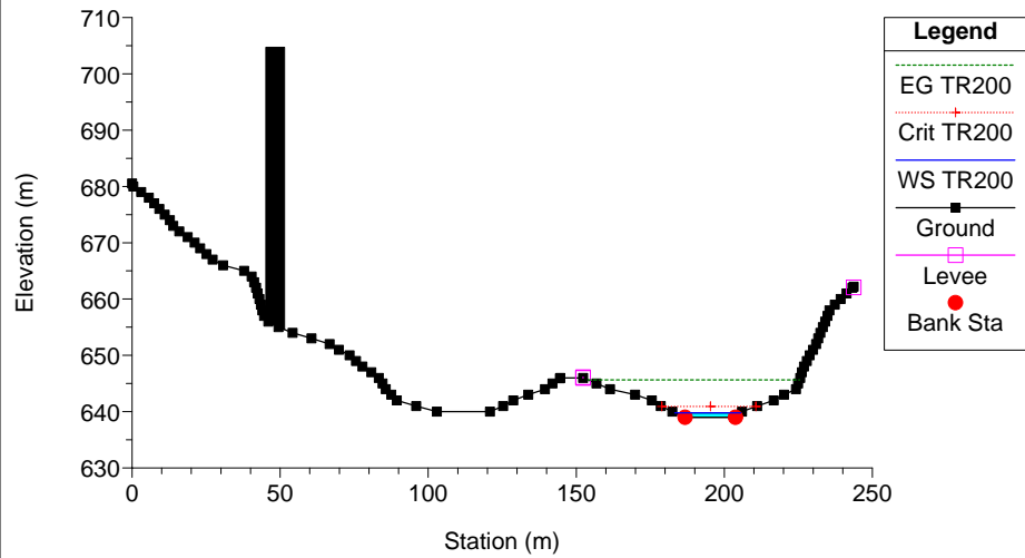
Clarea_Stato attuale Plan: Plan 08 21/01/2013 River = 6 Reach = 6 RS = 30
