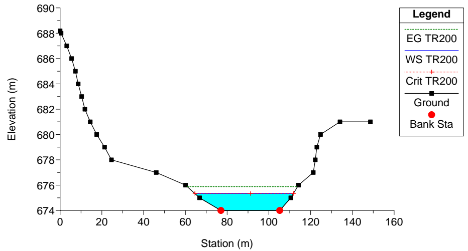
Clarea_Stato attuale Plan: Plan 08 21/01/2013 River = 6 Reach = 6 RS = 29
