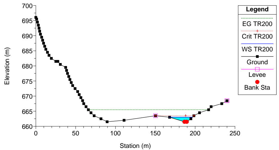
Clarea_Stato attuale Plan: Plan 08 21/01/2013 River = 6 Reach = 6 RS = 20
