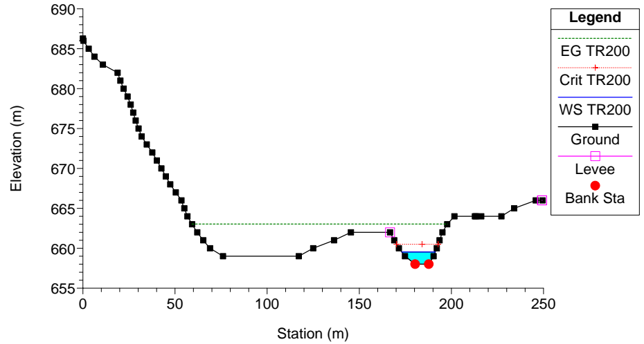
Clarea_Stato di Progetto_2 Plan: Plan 11 21/01/2013 River = 6 Reach = 6 RS = 15
