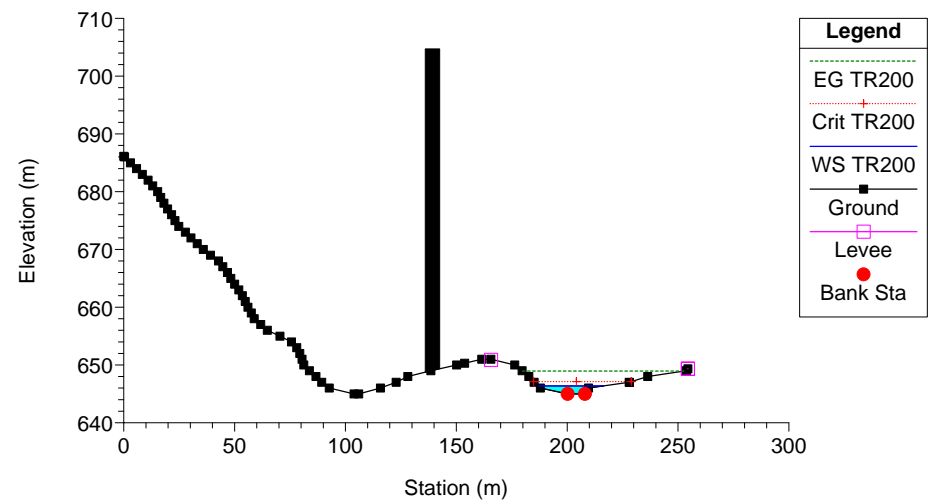
Clarea_Stato di Progetto_2 Plan: Plan 11 21/01/2013 River = 6 Reach = 6 RS = 3
