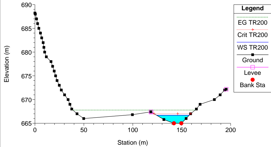
Clarea_Stato attuale Plan: Plan 08 21/01/2013 River = 6 Reach = 6 RS = 21
