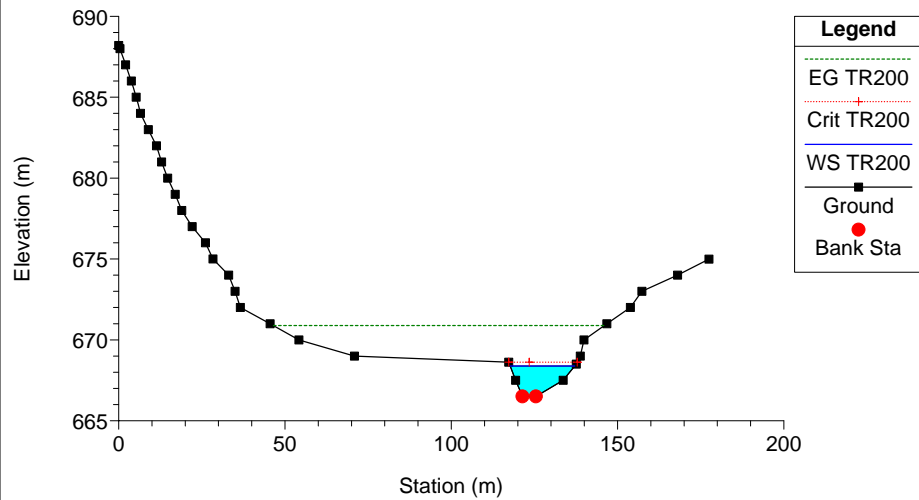
Clarea_Stato di Progetto_2 Plan: Plan 11 21/01/2013 River = 6 Reach = 6 RS = 26
