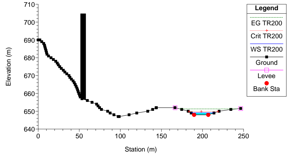
Clarea_Stato di Progetto_2 Plan: Plan 11 21/01/2013 River = 6 Reach = 6 RS = 3
