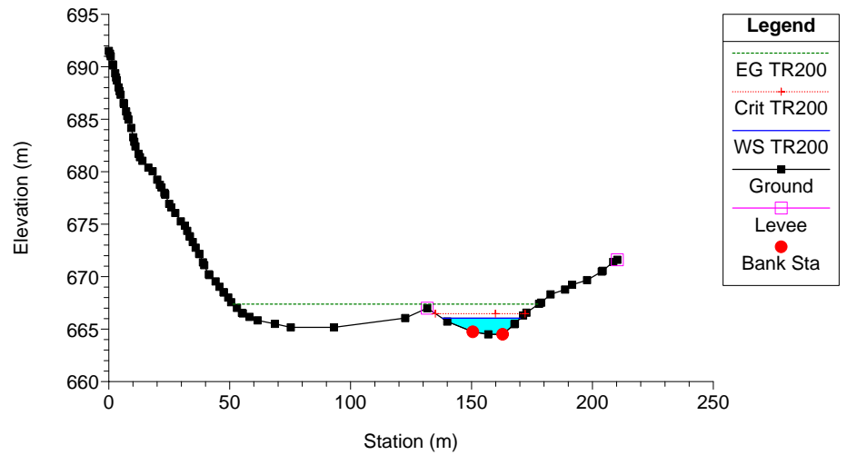
Clarea_Stato attuale Plan: Plan 08 21/01/2013 River = 6 Reach = 6 RS = 20
