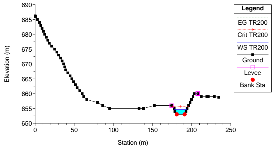
Clarea_Stato attuale Plan: Plan 08 21/01/2013 River = 6 Reach = 6 RS = 10
