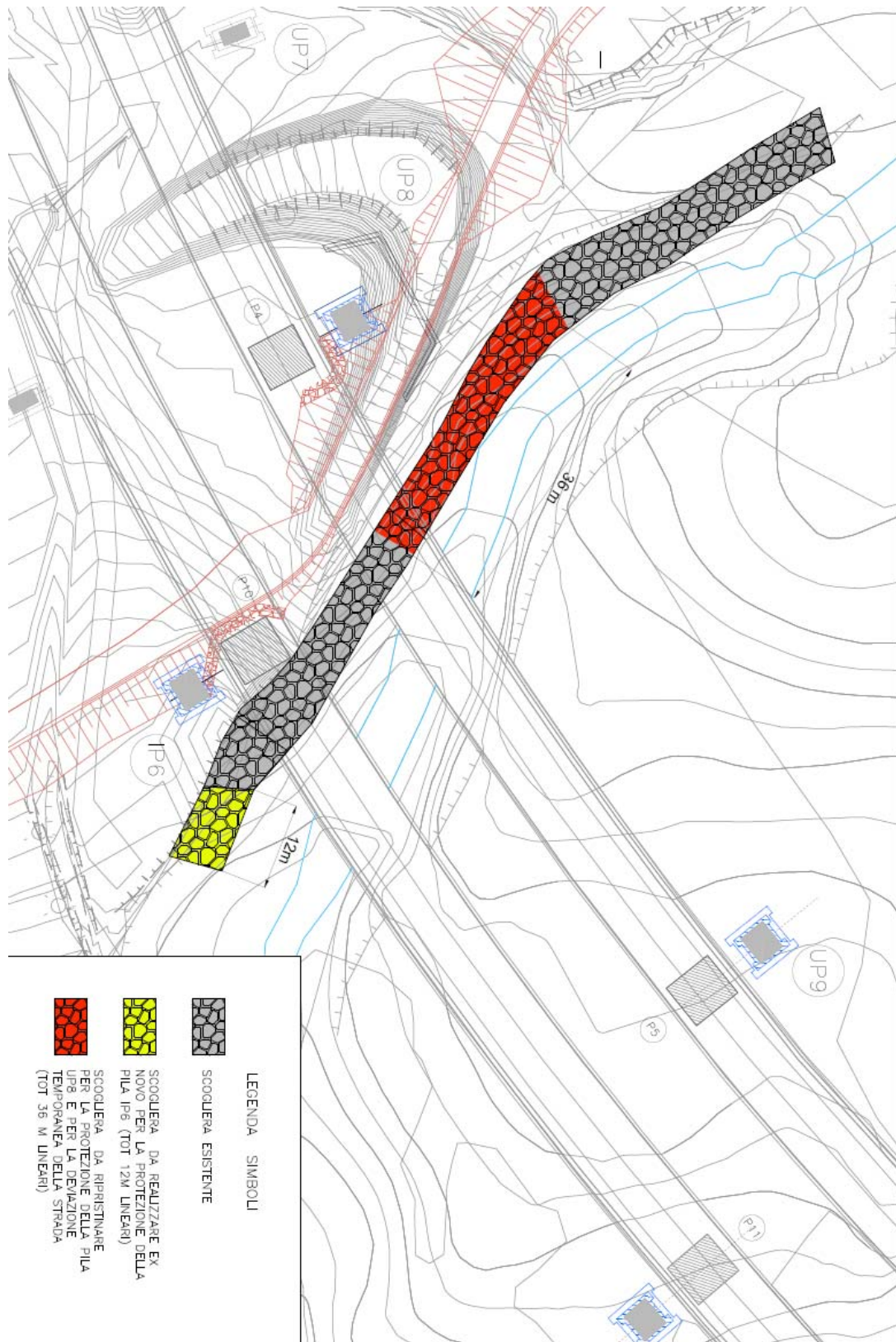
Fig. 20 – Planimetria realizzazione e ripristino scogliera protezione sponda
