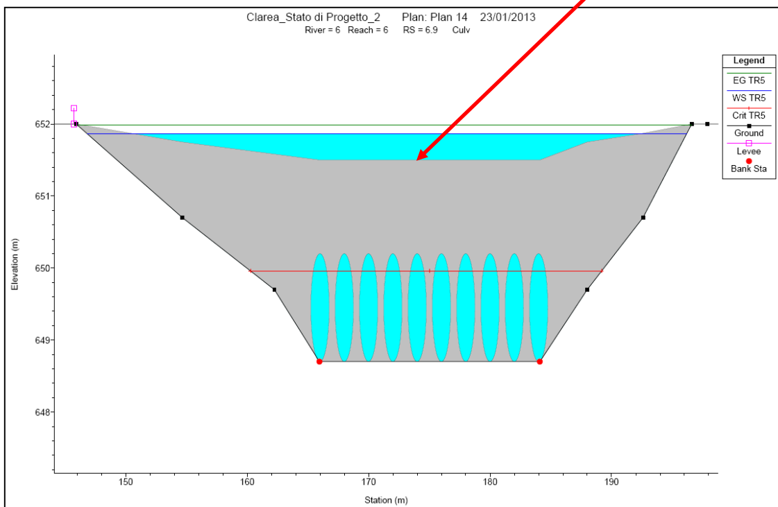
Fig. 24 – Sezione RS 6.9 Guado provvisorio
