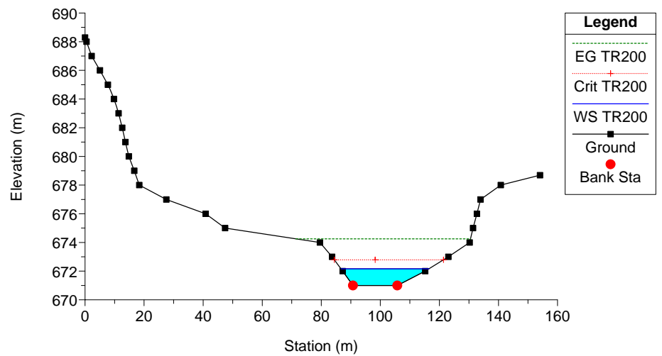
Clarea_Stato attuale Plan: Plan 08 21/01/2013 River = 6 Reach = 6 RS = 29
