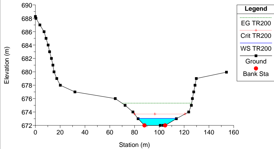
Clarea_Stato di Progetto_2 Plan: Plan 11 21/01/2013 River = 6 Reach = 6 RS = 30
