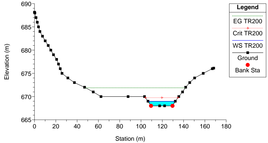
Clarea_Stato di Progetto_2 Plan: Plan 11 21/01/2013 River = 6 Reach = 6 RS = 24
