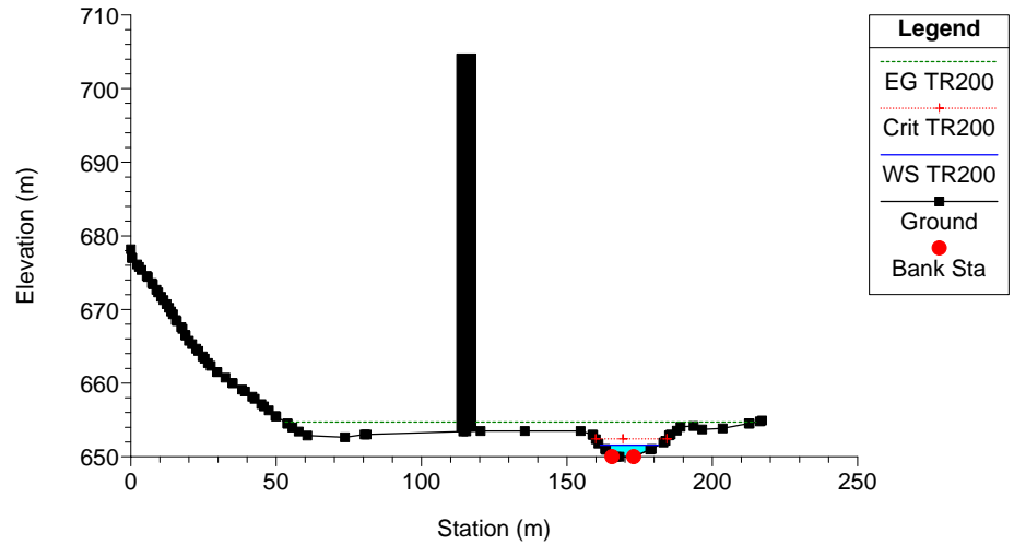
Clarea_Stato attuale Plan: Plan 08 21/01/2013 River = 6 Reach = 6 RS = 7
