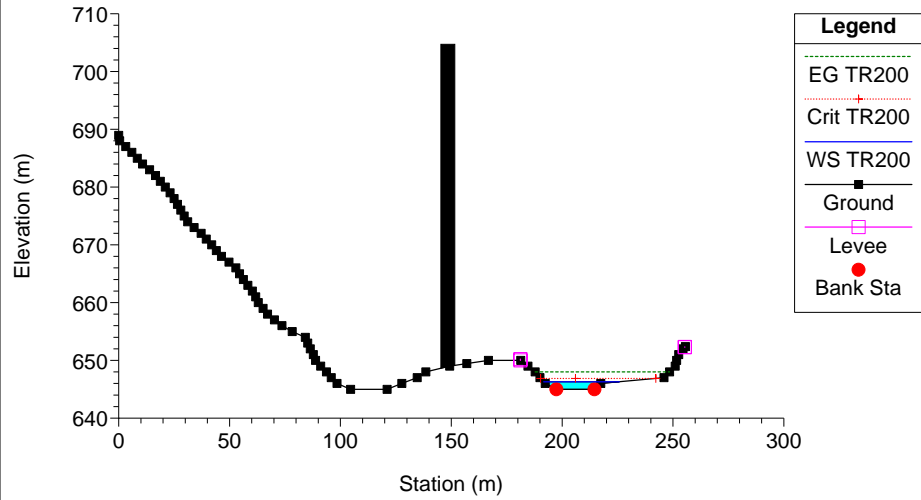
Clarea_Stato attuale Plan: Plan 08 21/01/2013 River = 6 Reach = 6 RS = 2
