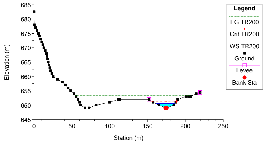
Clarea_Stato attuale Plan: Plan 08 21/01/2013 River = 6 Reach = 6 RS = 7
