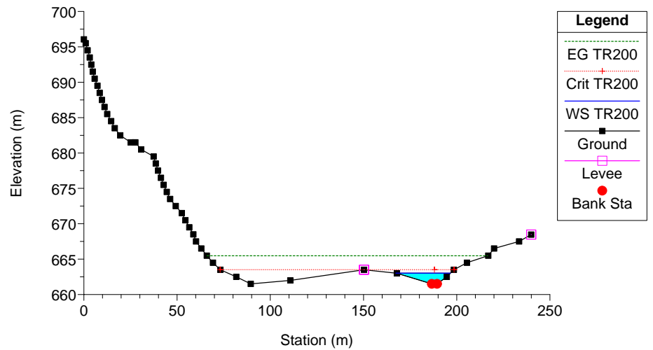
Clarea_Stato di Progetto_2 Plan: Plan 11 21/01/2013 River = 6 Reach = 6 RS = 20
