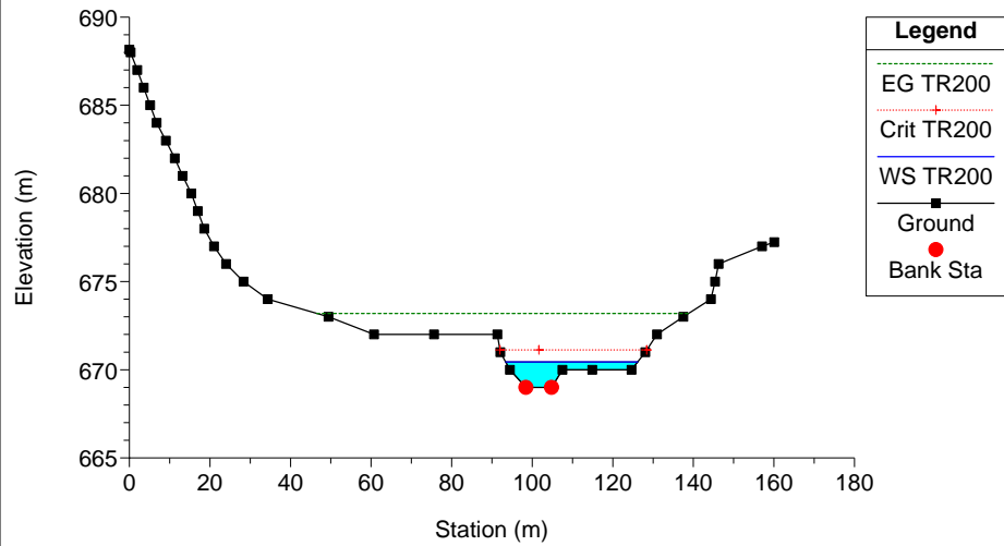
Clarea_Stato attuale Plan: Plan 08 21/01/2013 River = 6 Reach = 6 RS = 26
