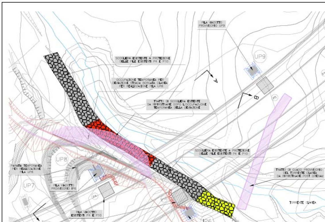
Fig. 8 – Opere provvisorie_ Deviazione viabilità esistente e Guado (in lilla)
