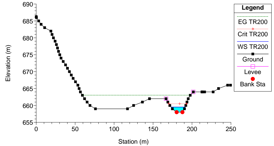
Clarea_Stato attuale Plan: Plan 08 21/01/2013 River = 6 Reach = 6 RS = 15
