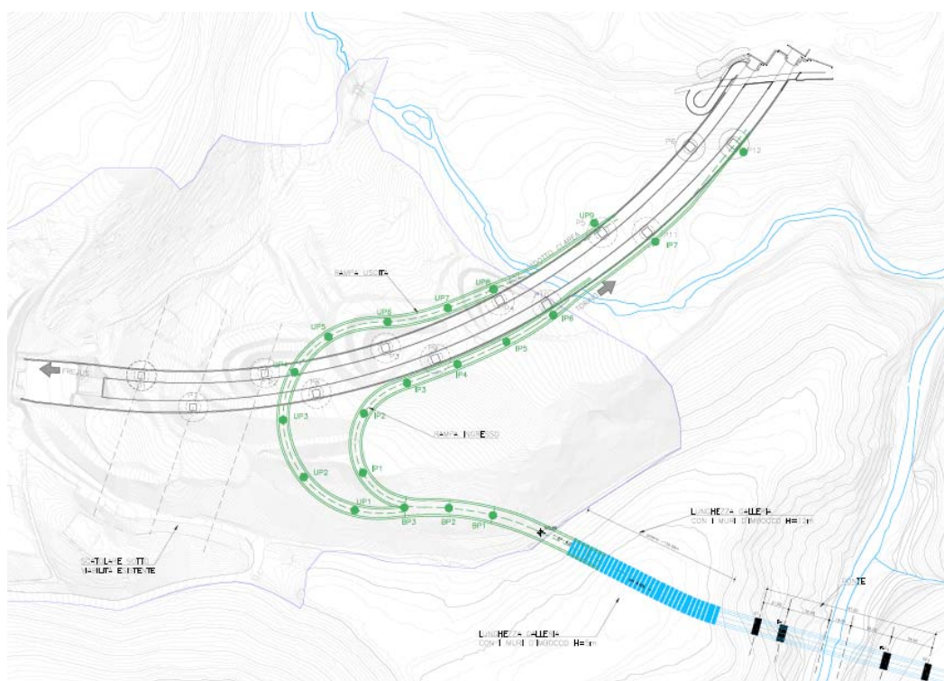
Fig. 6 –Svincolo sulla A32
