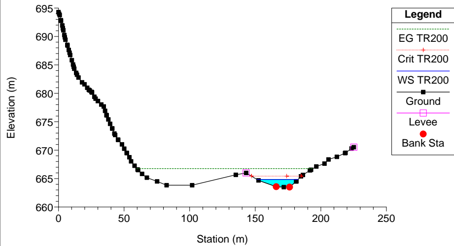
Clarea_Stato di Progetto_2 Plan: Plan 11 21/01/2013 River = 6 Reach = 6 RS = 21
