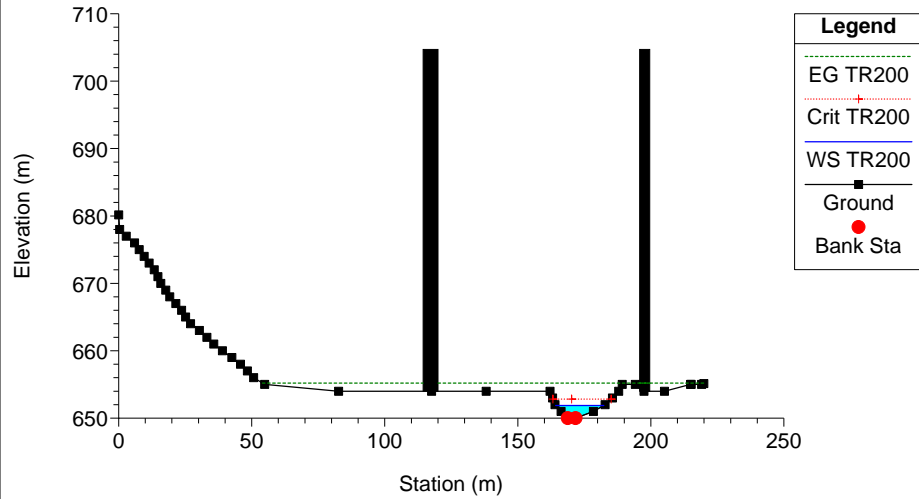
Clarea_Stato di Progetto_2 Plan: Plan 11 21/01/2013 River = 6 Reach = 6 RS = 8
