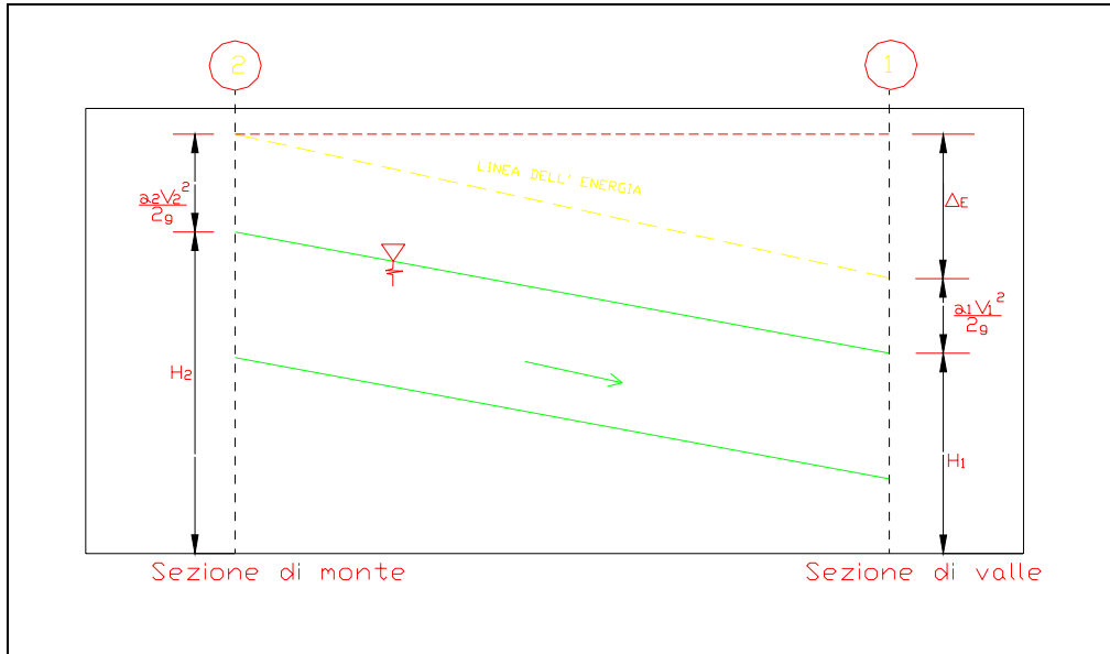
Figura 12: Grandezze presenti nell'equazione dell'energia.
