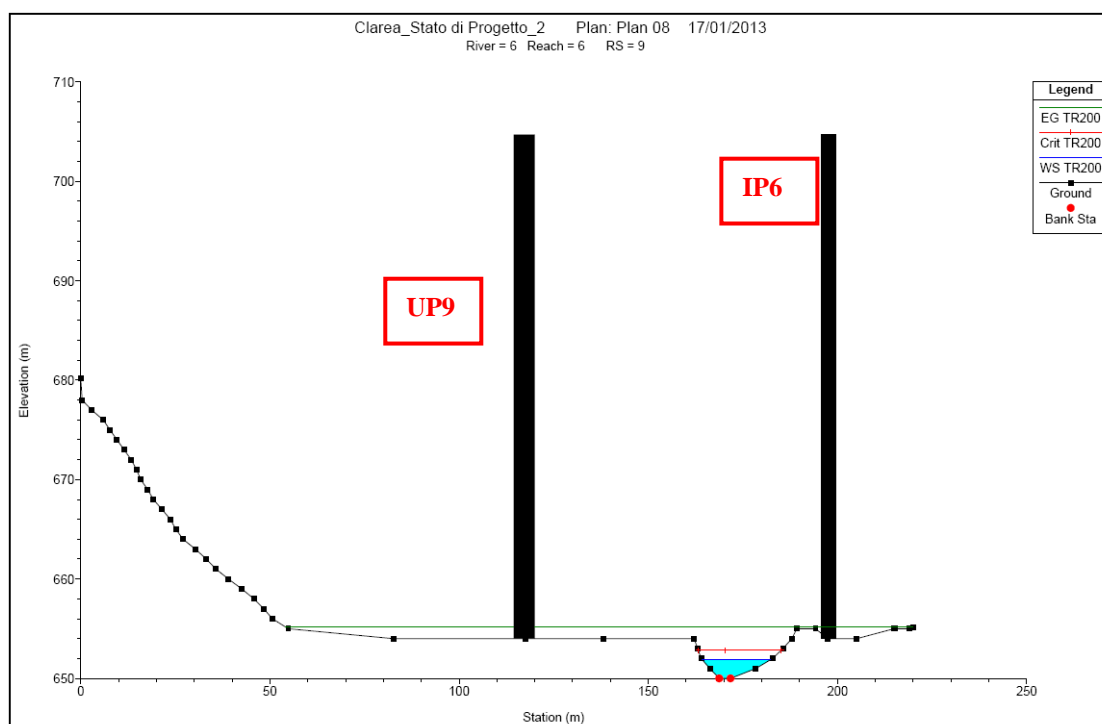
Fig. 18 – Sezione idraulica RS10
