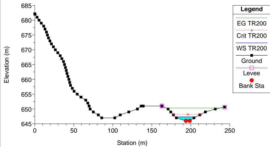
Clarea_Stato attuale Plan: Plan 08 21/01/2013 River = 6 Reach = 6 RS = 4
