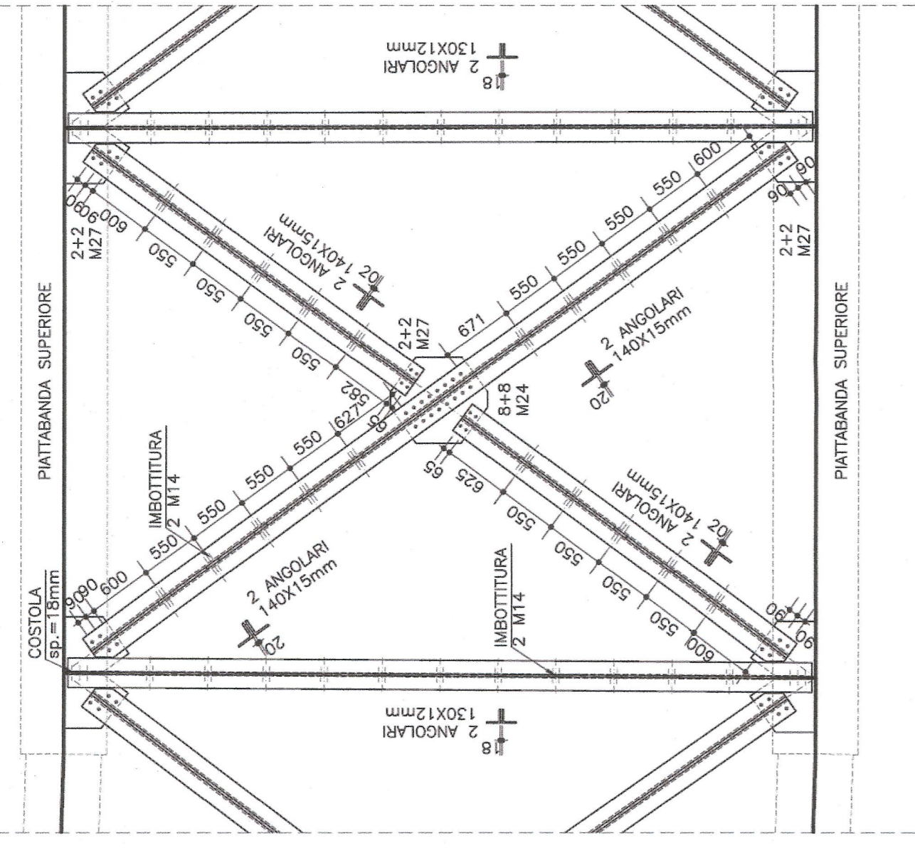
DIAGONALI DI CONTROVENTAMENTO SUPERIORI BP2-BP3 PIANTA scala 1:50
