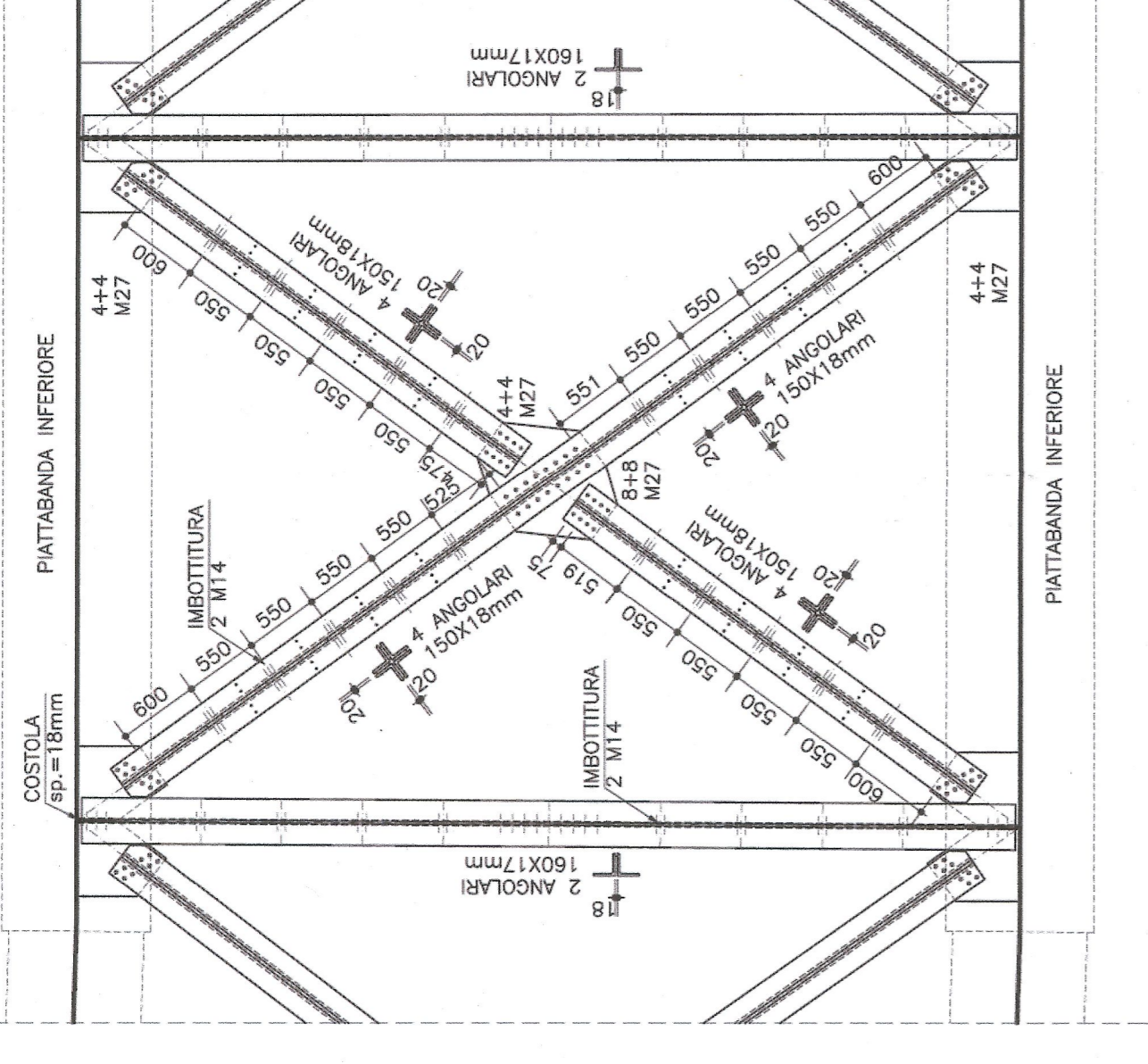
DIAGONALI DI CONTROVENTAMENTO INFERIORI BP2-BP3 PIANTA scala 1:50
