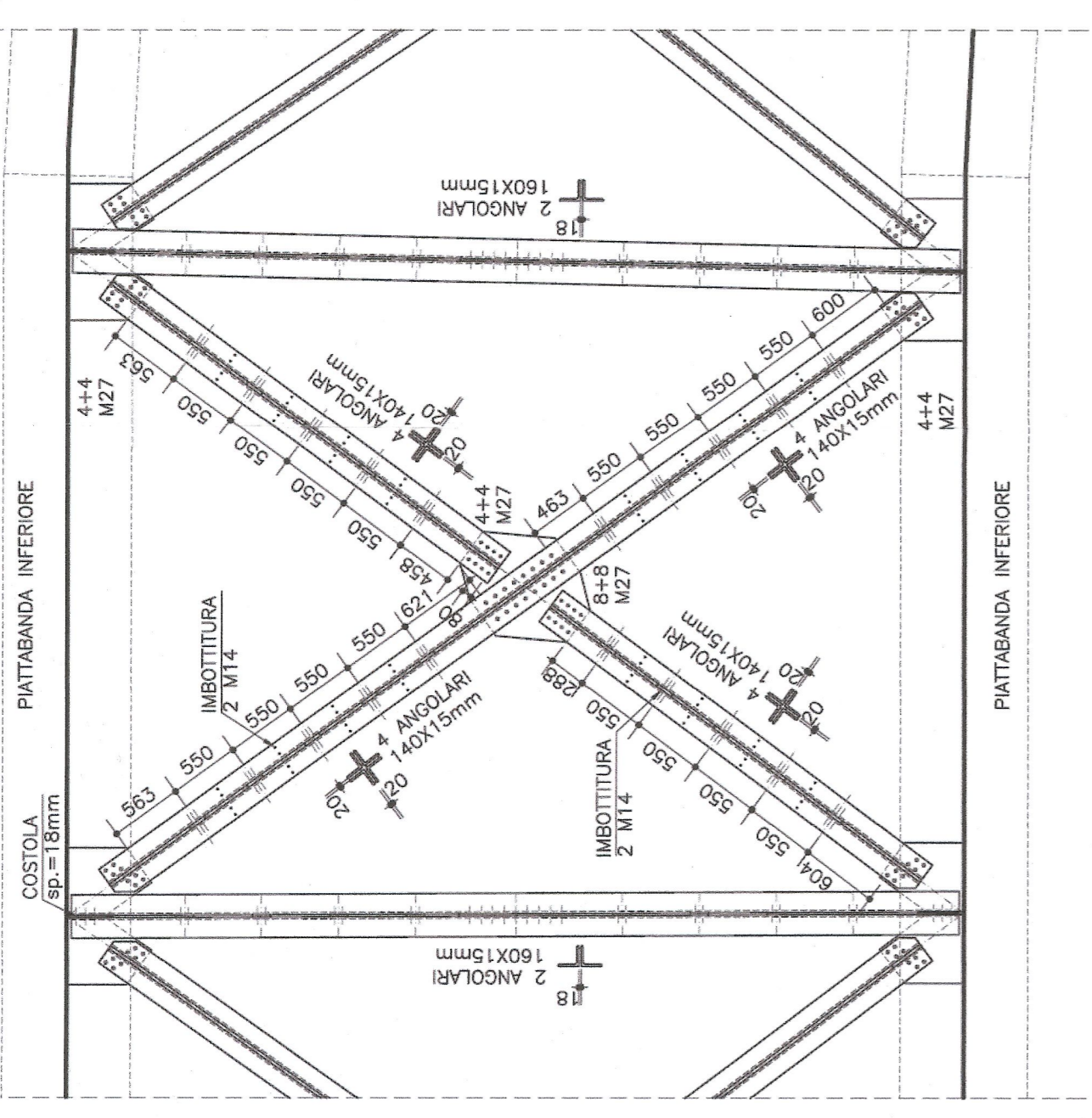
DIAGONALI DI CONTROVENTAMENTO INFERIORI BP1-BP2 PIANTA scala 1:50
