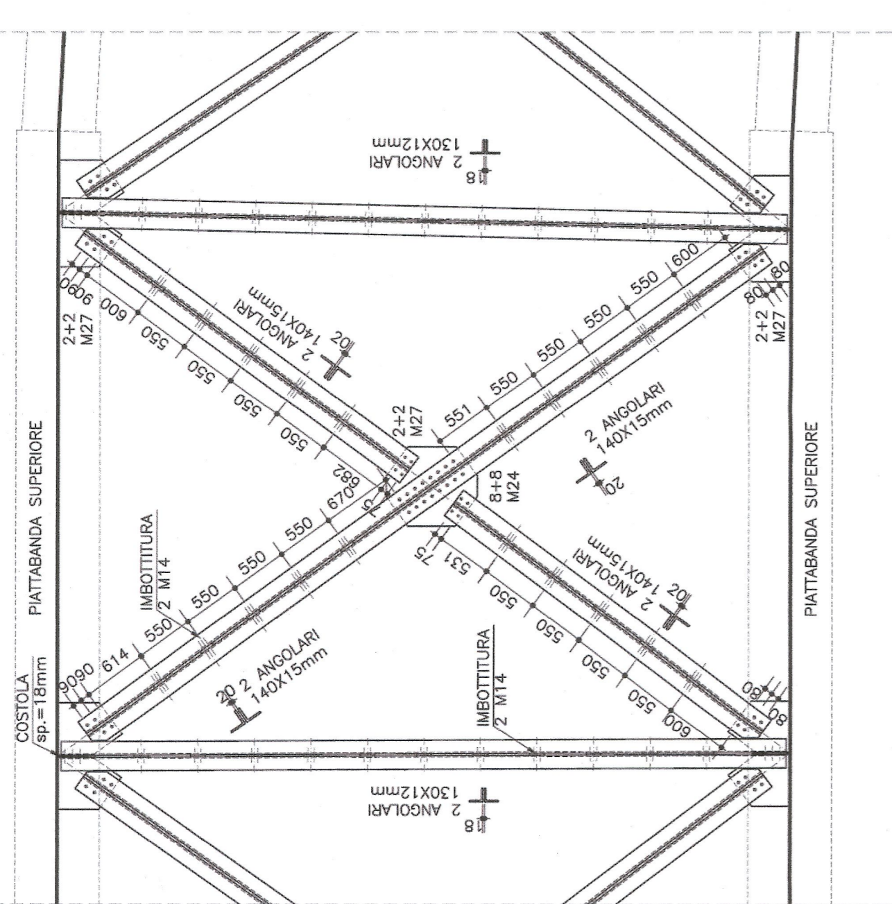
DIAGONALI DI CONTROVENTAMENTO SUPERIORI BP1-BP2 PIANTA scala 1:50
