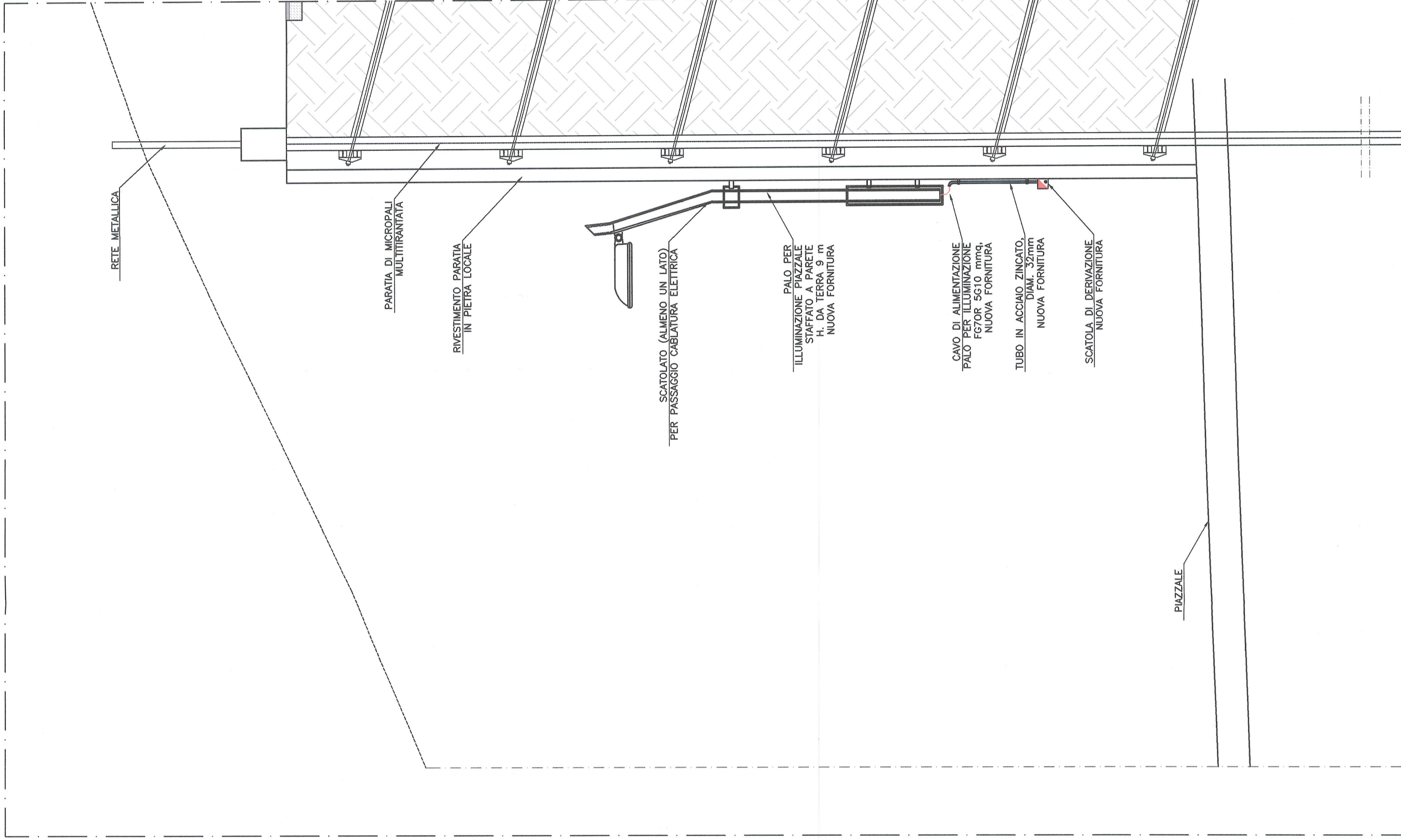
SEZIONE C-C SEZIONE TIPO PIAZZALE - STATO IN PROGETTO scala 1:50
