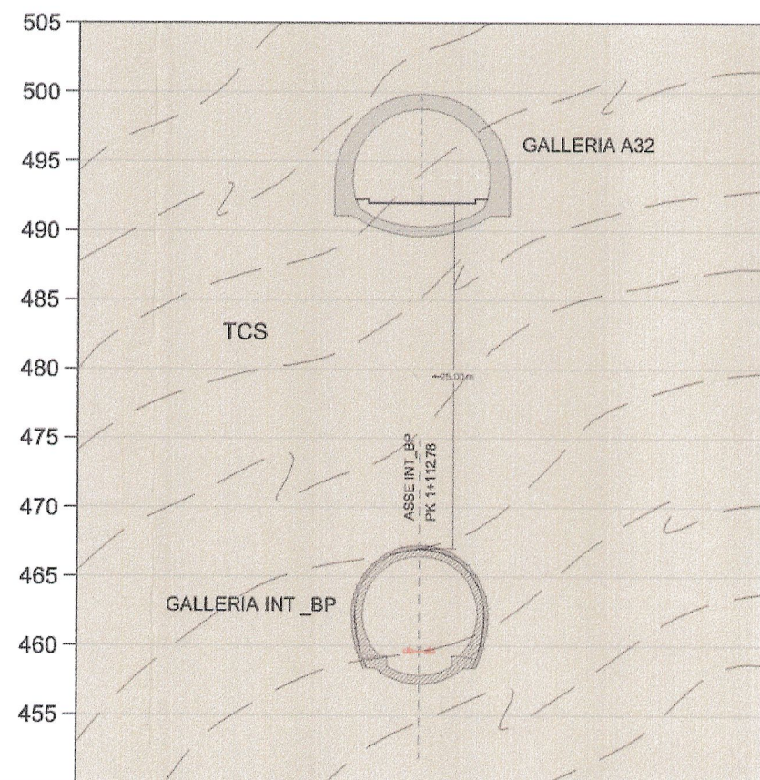
Sezione / Section V1-V2 Interferenza INT_BP - A32 scala / échelle 1:500/500
