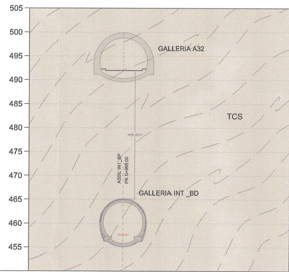
Sezione / Section U1-U2 Interferenza INT_BP - A32 scala / échelle 1:500/500
