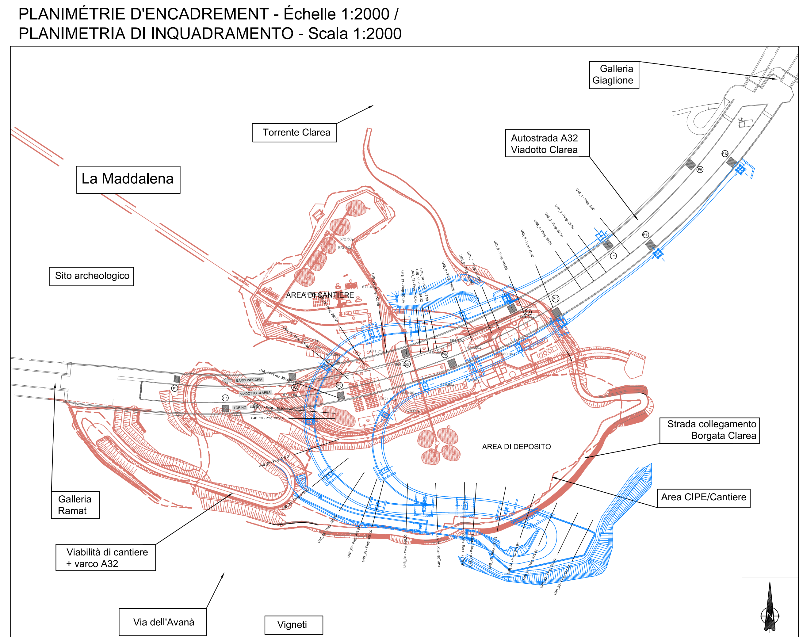
PLANIMÉTRIE D'ENCADREMENT - Échelle 1:2000 / PLANIMETRIA DI INQUADRAMENTO - Scala 1:2000
