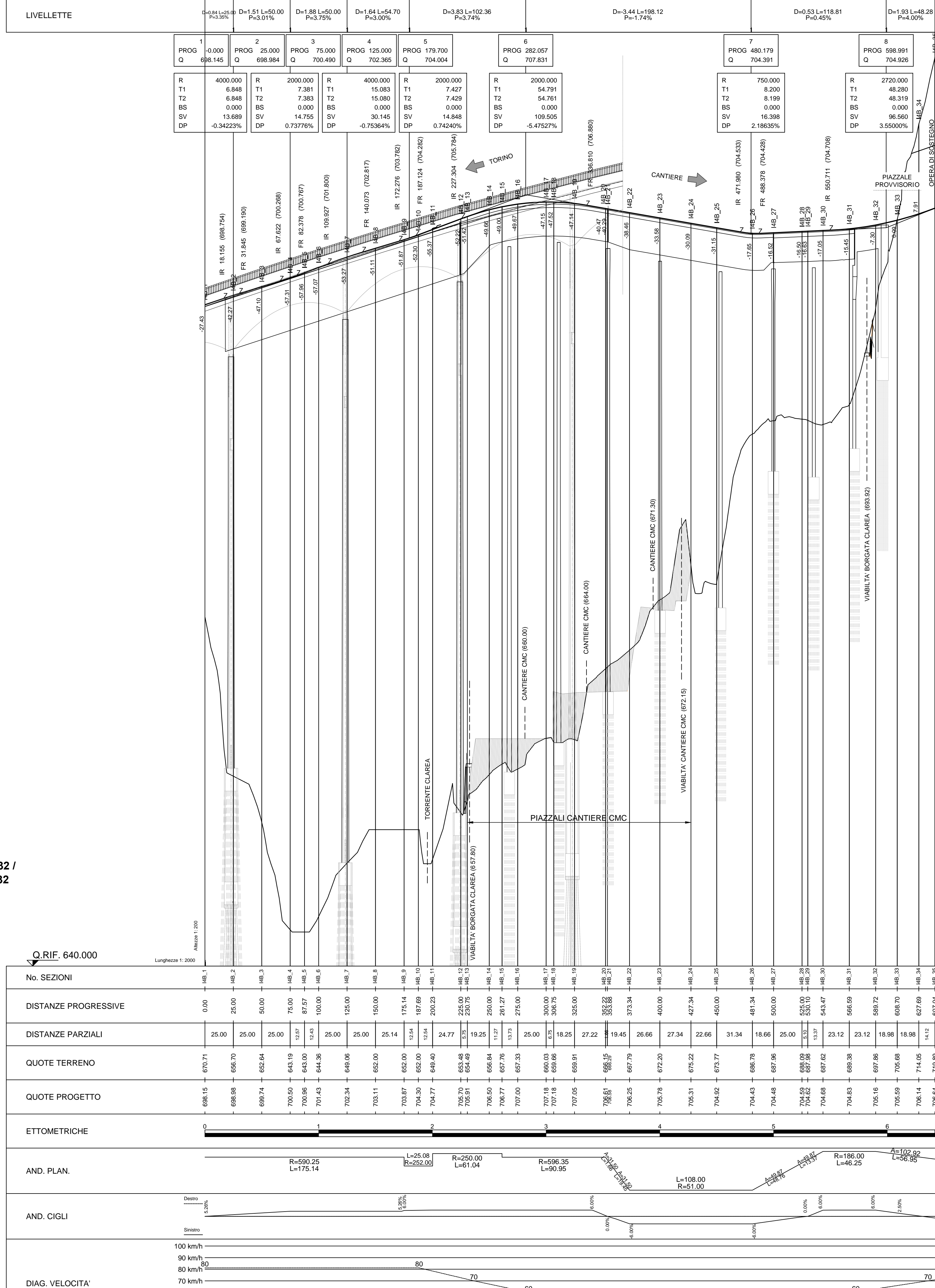
RAMPE D'ENTRÉE SUR LA A32 / RAMPA DI INGRESSO SULLA A32
